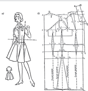
Рис. 170. Нарядное платье: а — общий вид; б — детали выкройки.
